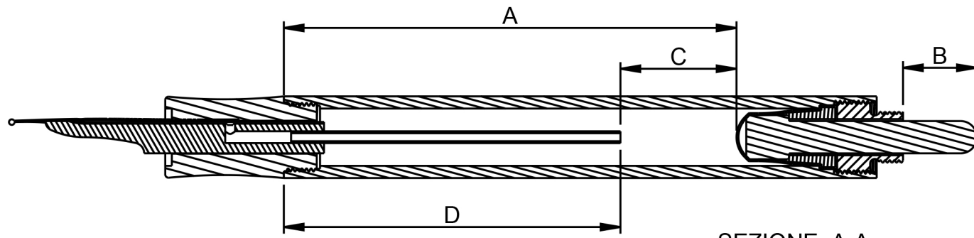
SEZIONE A-A
